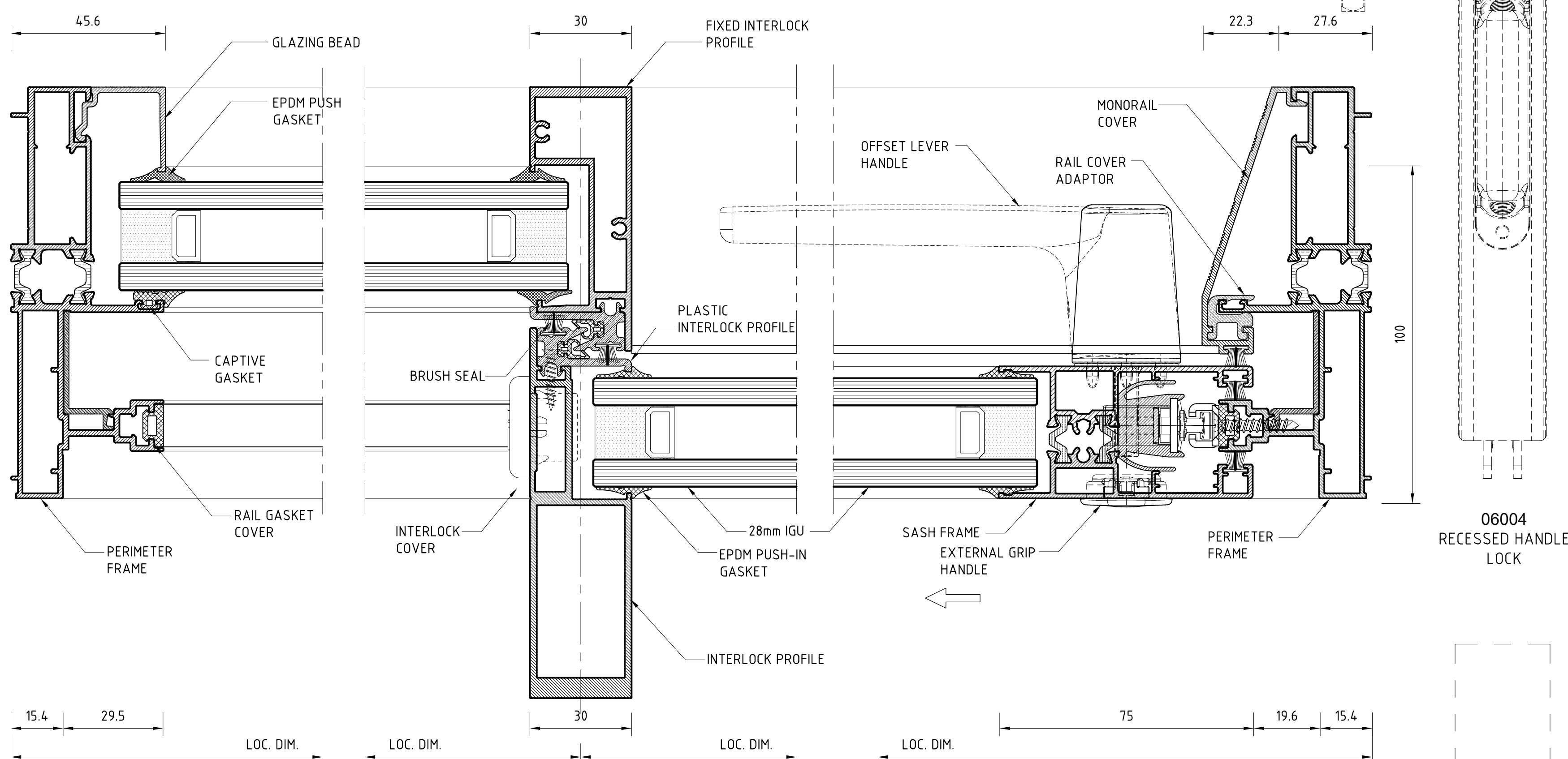
JAMB DETAIL
